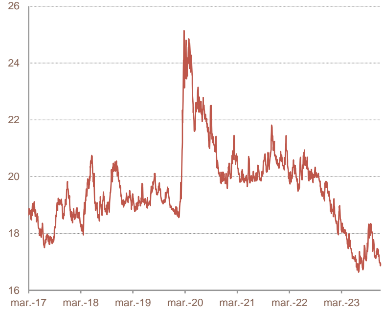
USDMXN
